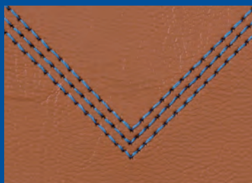
Vitesse de couture : 2 800 points/min, longueur de point : 4 mm
